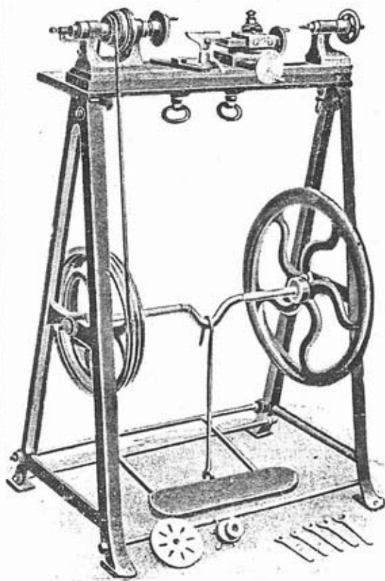
Šlapací soustruh
